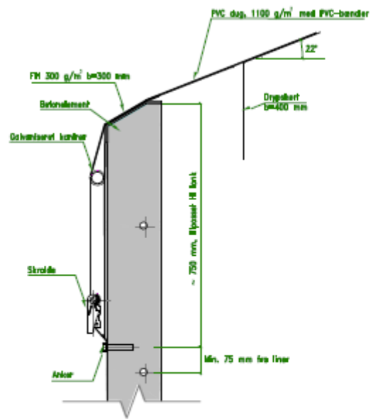
DETALJE A
