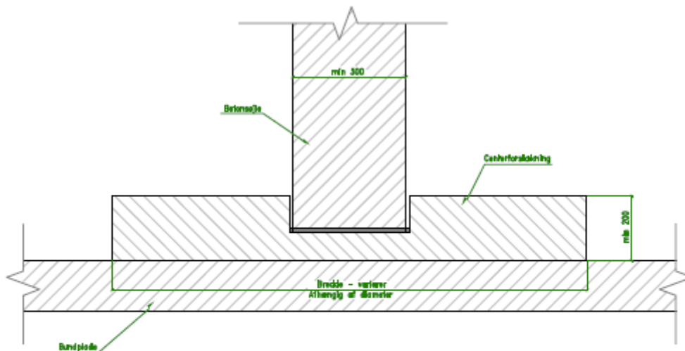
DETALJE B
